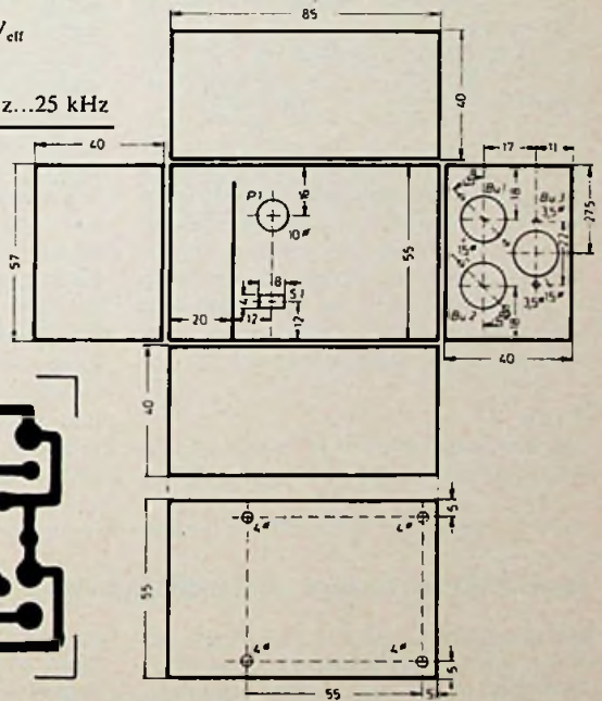
Fig. 6. Samenstelling van het kastje.
